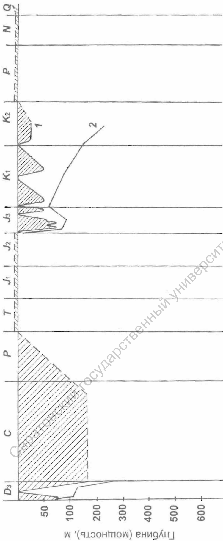
Рис. 4. Графики палеогеографической и эпейрогенетической кривых: 1 – палеогеографическая кривая; 2 – эпейрогенетическая кривая
